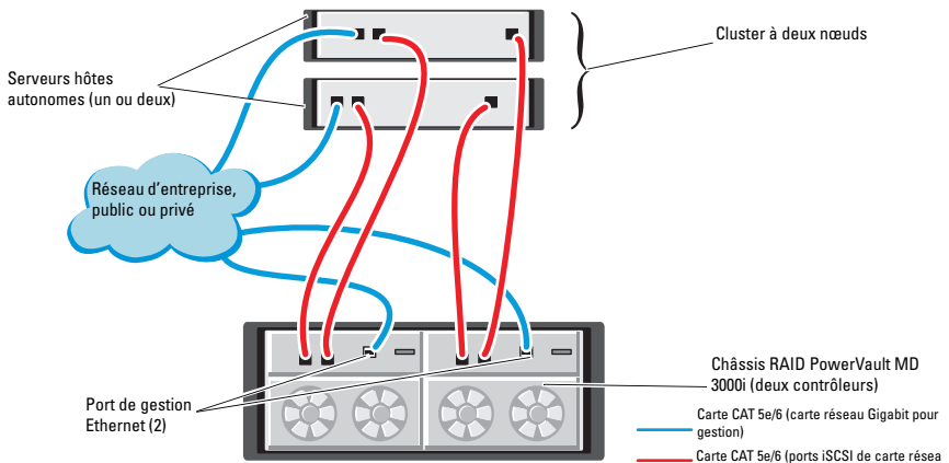
Figure 4-1. Câblage de clusters iSCSI à connexion directe
