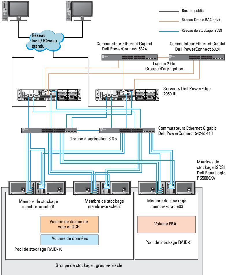
Figure 5-2. Exemple de configuration Oracle RAC à trois matrices PS5000XV
