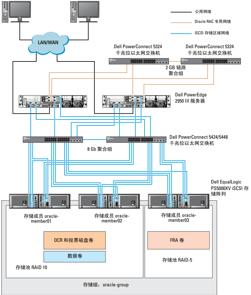
图 5-2. 使用三个 PS5000XV 阵列的 Oracle RAC 配置示例
