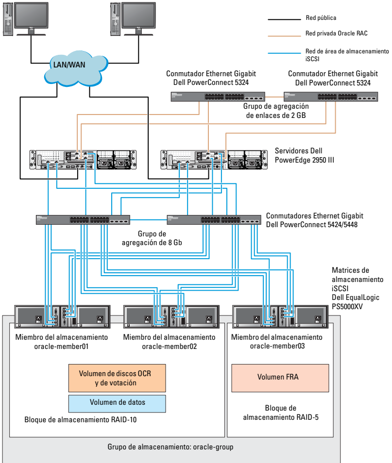
Ilustración 5-2. Configuración de Oracle RAC de muestra con tres matrices PS5000XV
