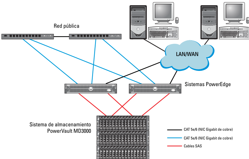
Ilustración 3-1. Cableado del clúster SCSI de conexión serie (SAS) y Dell PowerVault MD3000
