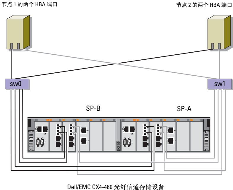
图 2-2. 在 Dell/EMC SAN 连接的光纤信道群集中布线
