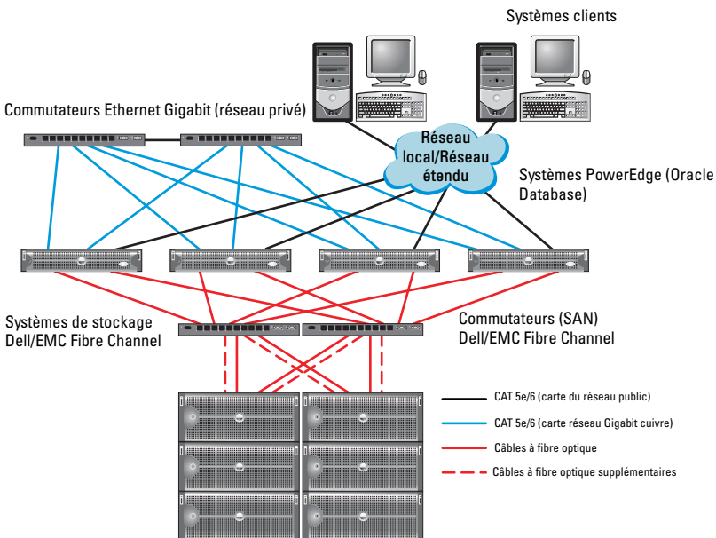
Figure 2-1. Connexions matérielles pour un cluster Fibre Channel connecté à un SAN
