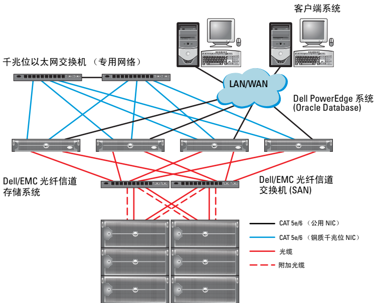
图 2-1. SAN 连接光纤信道群集的硬件连接
