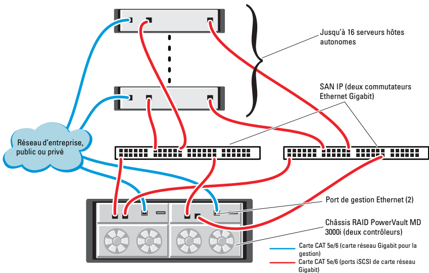
Figure 4-2. Câblage des clusters iSCSI avec liaison par commutateur
