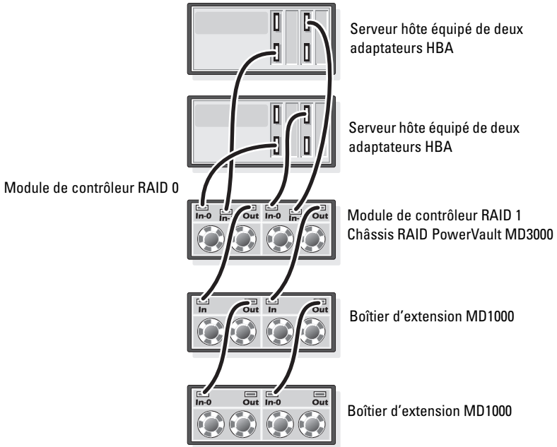
Figure 3-2. Câblage d'un cluster SAS à connexion directe
