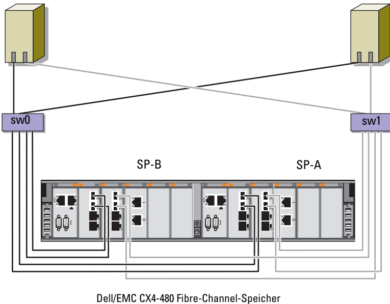
Abbildung 2-2. Dell/EMC SAN-Attach-Fibre-Channel-Cluster verkabeln
