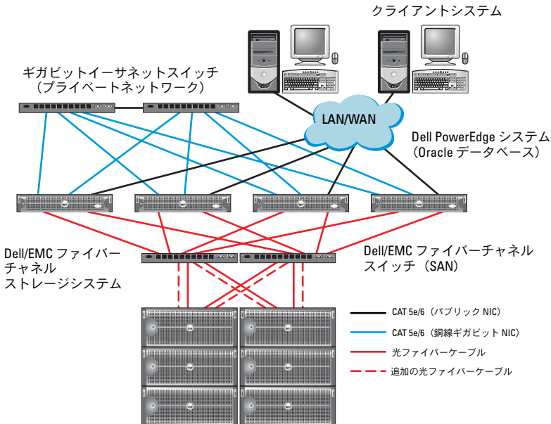
図 2-1 SAN 接続のファイバーチャネルクラスタ用のハードウェア接続
