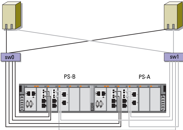
Figure 2-2. Câblage d'un cluster Fibre Channel Dell/EMC connecté à un réseau de stockage (SAN)
