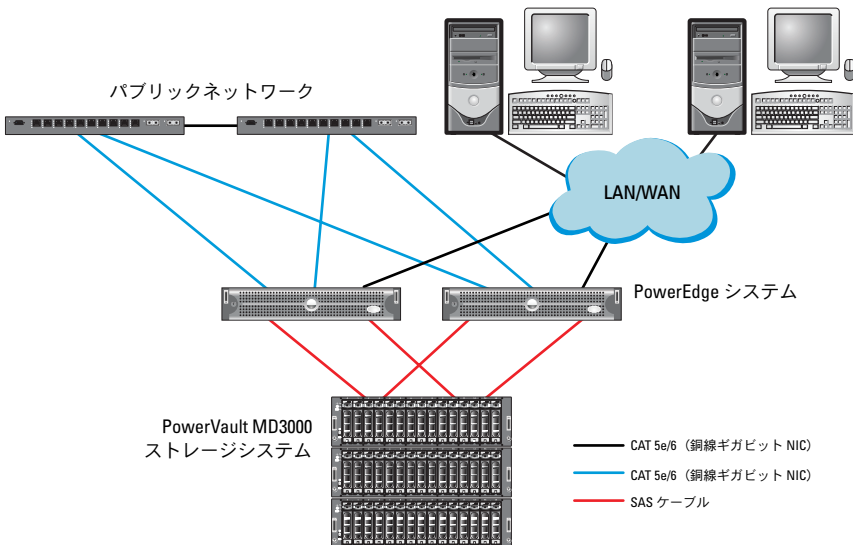
図 3-1 SAS（シリアル接続 SCSI）クラスターと Dell PowerVault MD3000 のケーブル接続
