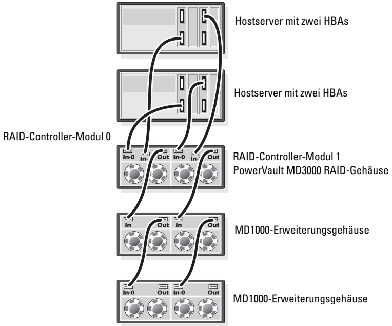
Abbildung 3-2. Direkt verbundenen SAS-Cluster verkabeln
